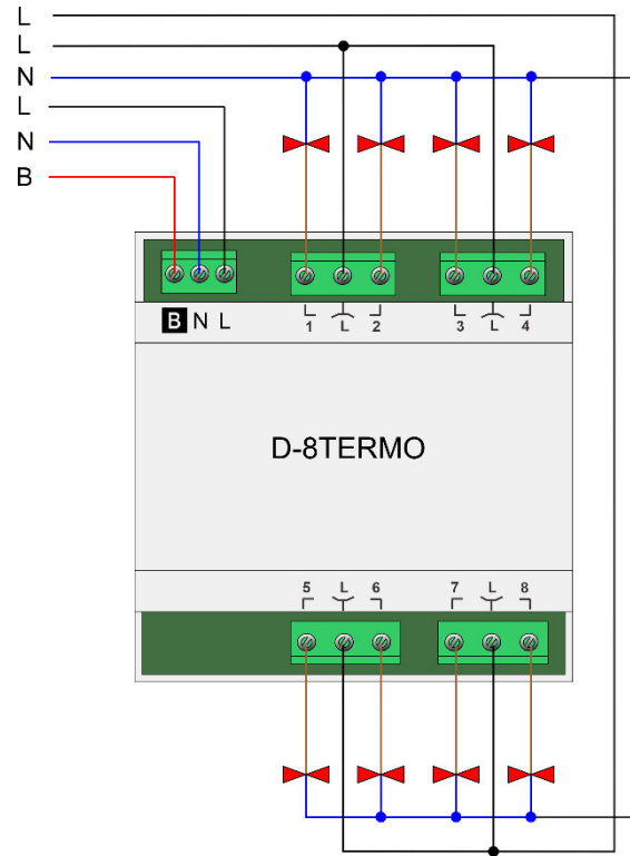
Esquema de Ligação:
